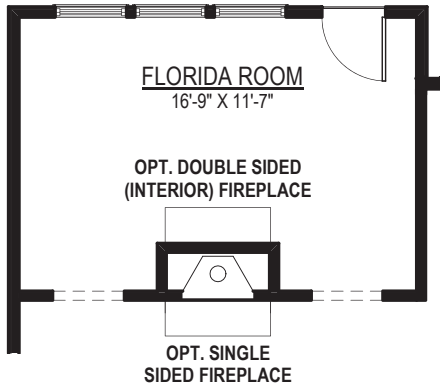
OPT. FLORIDA ROOM IN LIEU OF DECK
